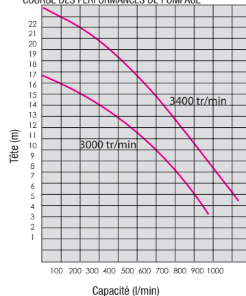
COURBE DES PERFORMANCES DE POMPAGE
